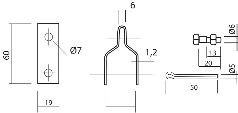
GANCHO MN89
