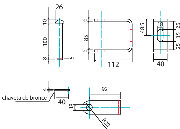
Rack - Soporte para aisladores roldana MN482 (para 1 aisladores)
