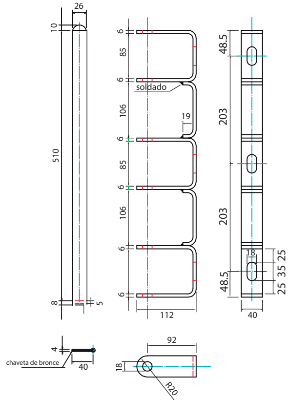
Rack - Soporte para aisladores roldana MN480 (para 3 aisladores)
