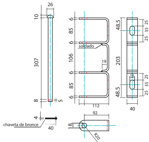
Rack - Soporte para aisladores roldana MN481 (para 2 aisladores)
