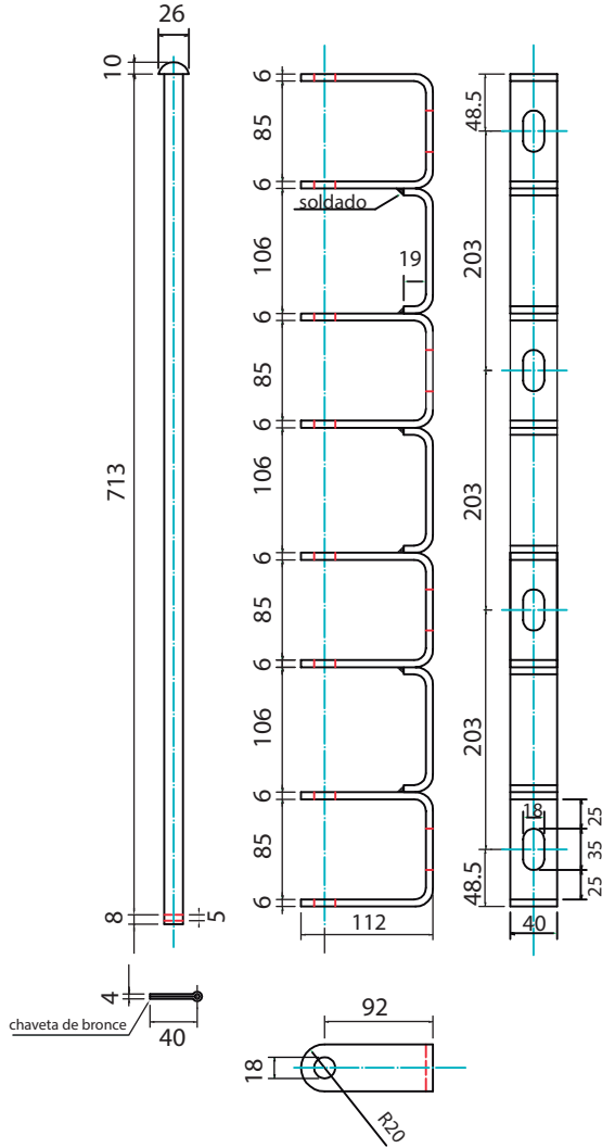
Rack - Soporte para aisladores roldana MN479 (para 4 aisladores)
