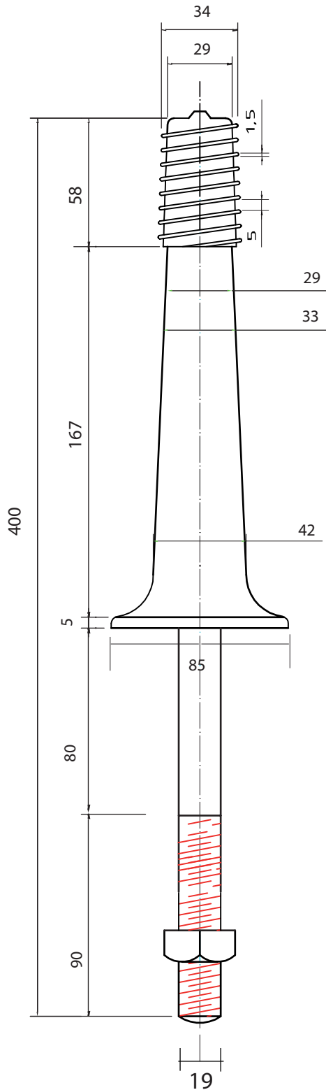
PERNO MN414
